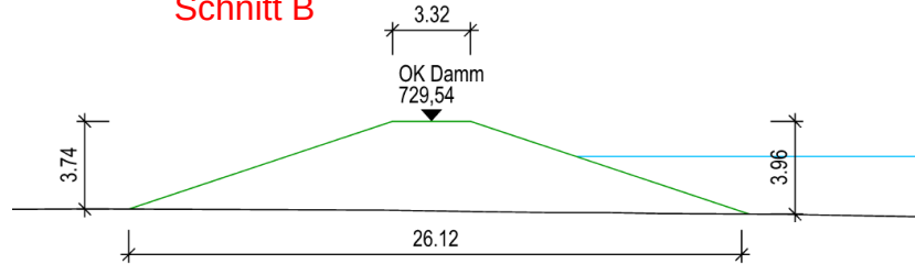
Schnitt B
