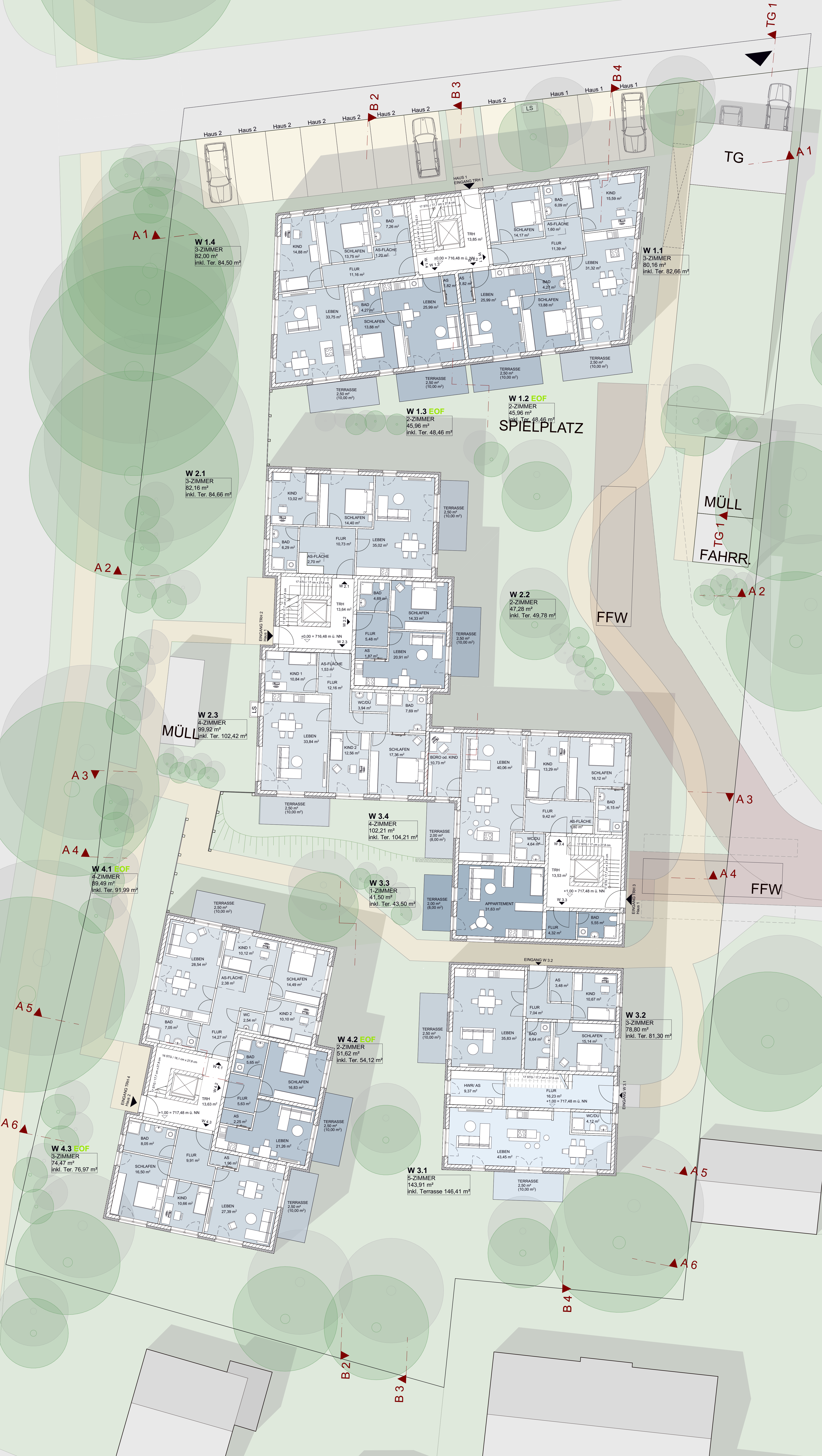
ERDGESCHOSS - M : 1 : 100
