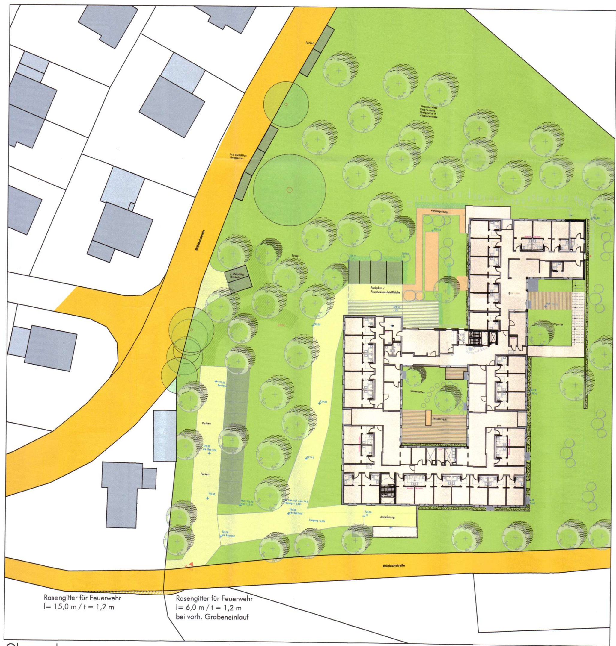
Obergeschoss
