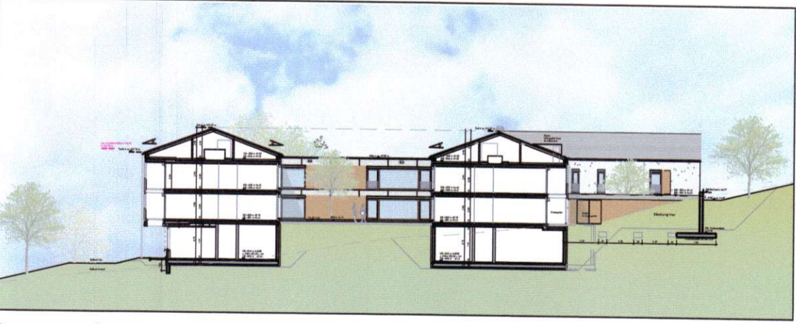
Systemschnitt
