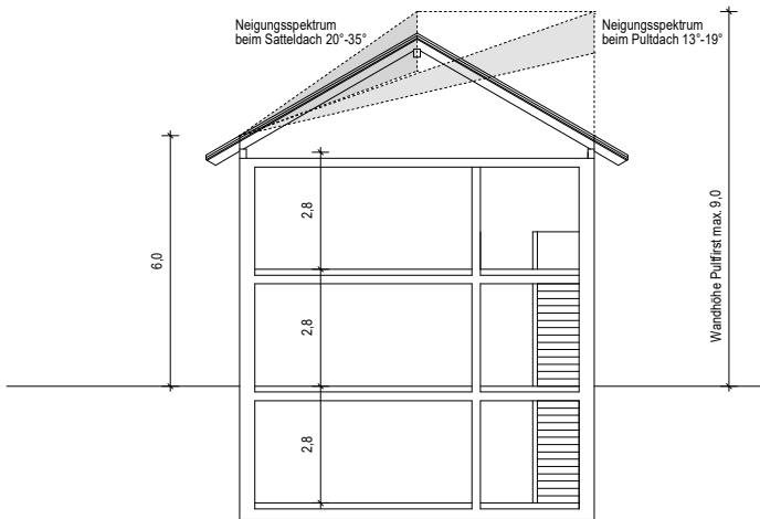
Regelschnitt Doppelhaus WA 1
